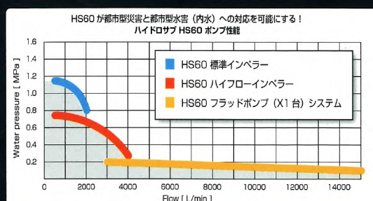
HS60 フラッドポンプ ×1 台 吐水圧 0.2MPa・毎分 15,000ℓ まで排水可能
