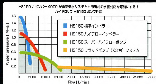
HS150 フラッドポンプ ×3 台 吐水圧 0.2MPa・毎分 45,000ℓ まで排水可能
